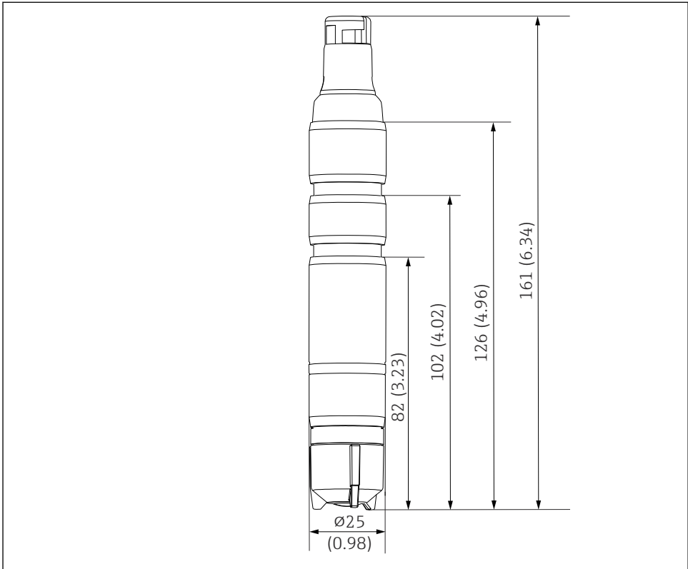
图 4 外形尺寸示意图；单位：mm (in)
