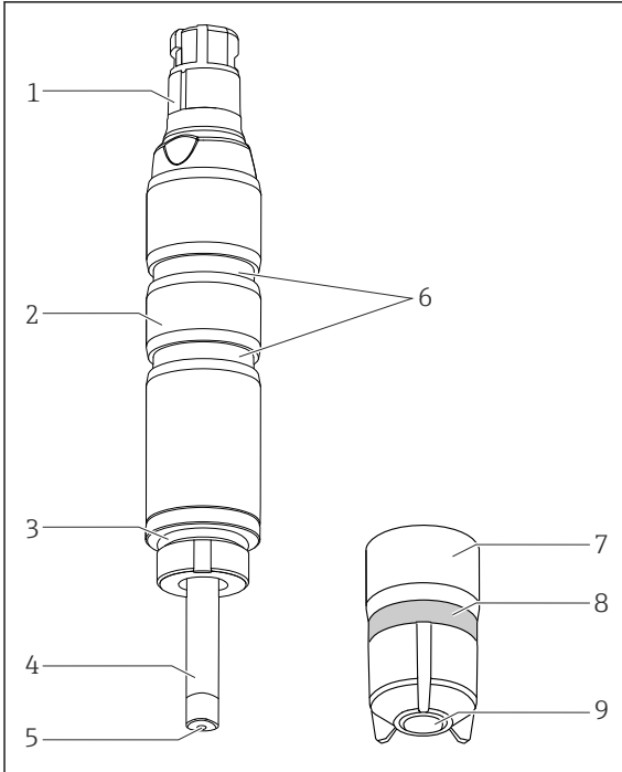
图 1 传感器结构
