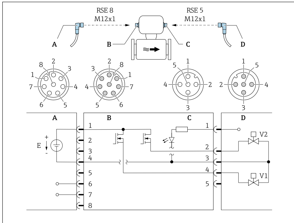
图 5 连接仪表
