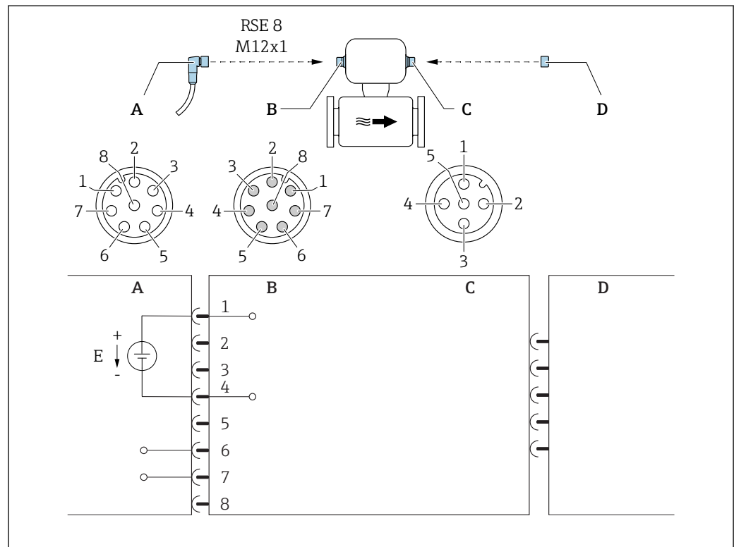
图 6 连接仪表
