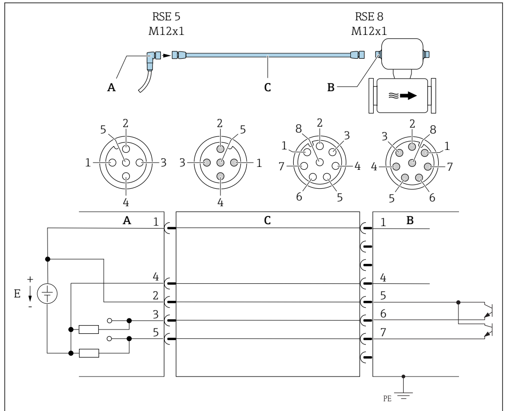
图 7 连接仪表
