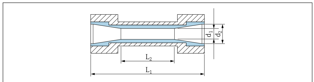
14 测量管的外形尺寸
