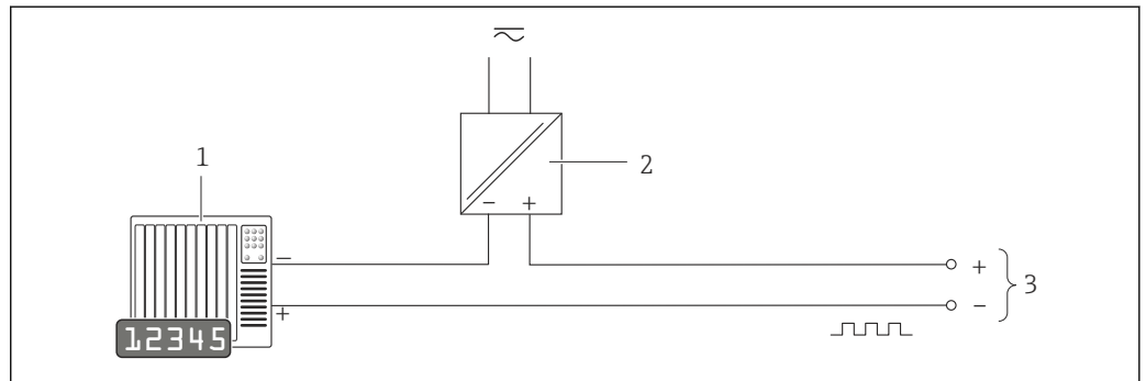
图 8 脉冲/频率输出(无源信号)的连接实例
