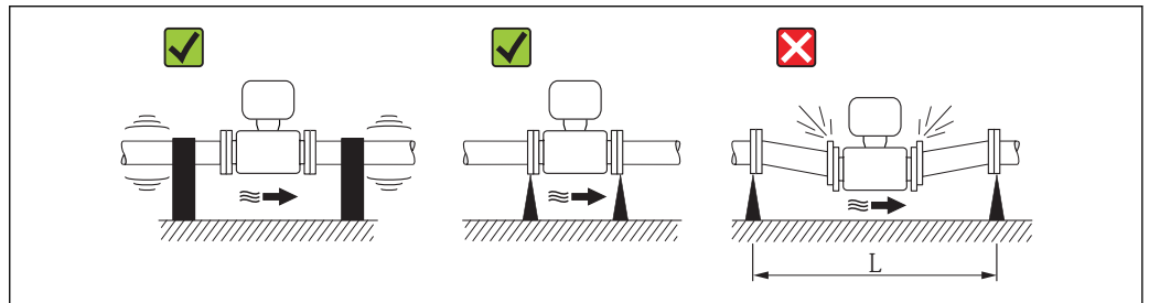
图 24 避免设备振动的措施(L > 10 m (33 ft))
