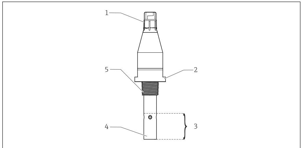
图 7 传感器结构
