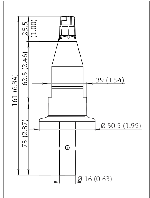
图 9 卡箍连接型
