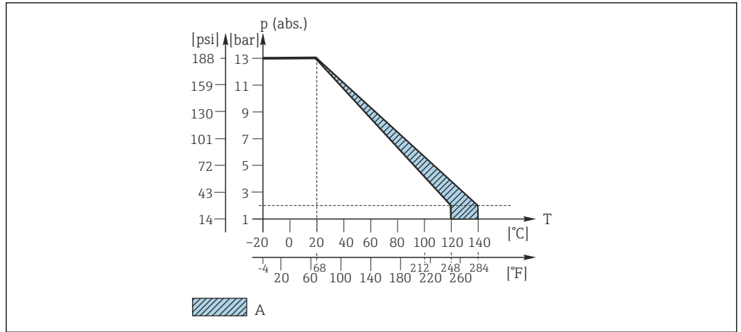
图 6 温压曲线
