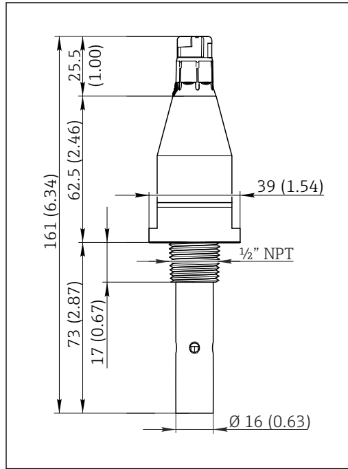
图 8 螺纹连接型
