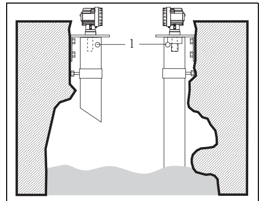
1 通风孔
