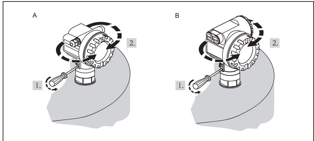
A F12 外壳
