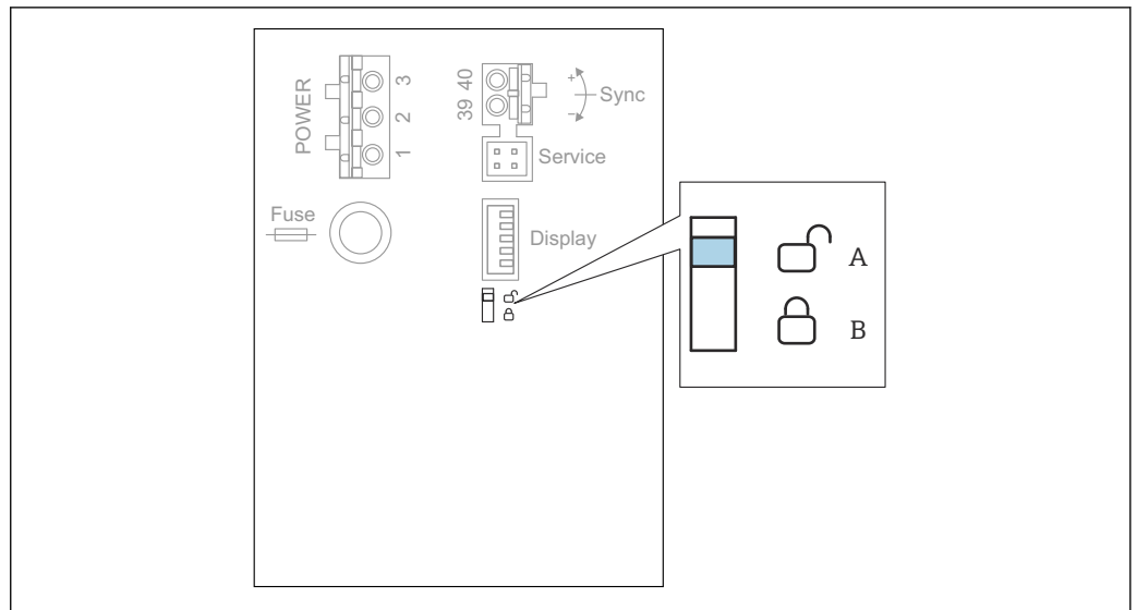
图 70 硬件锁定
