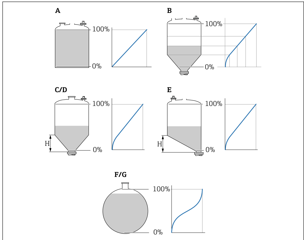
48 线性化类型
