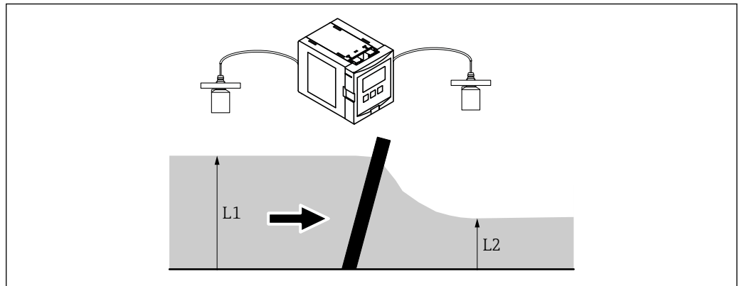
图 65 隔栅控制功能的工作原理
