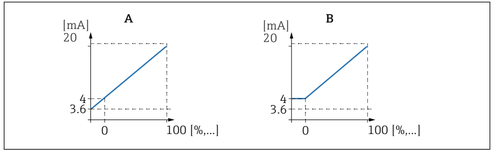
68 4mA 阈值 (仅当电流范围= 4 ... 20 mA)
