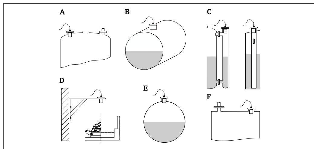
图 46 罐体形状
