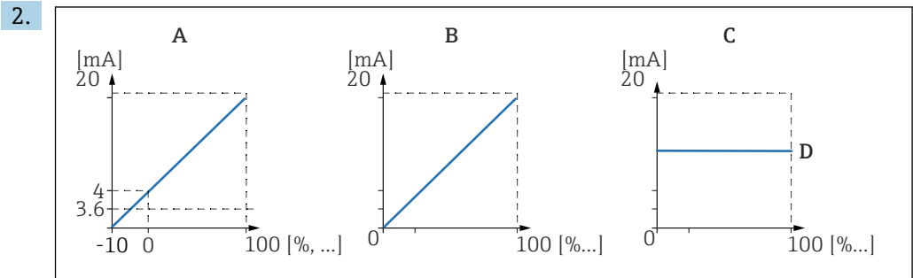
图 66 电流范围
