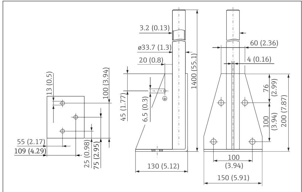
图 75 外形尺寸示意图。测量单位 mm (in)
