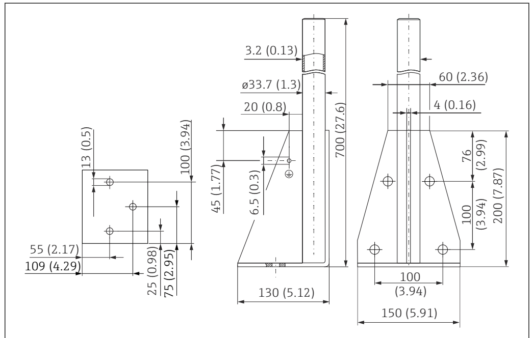
图 74 外形尺寸示意图。测量单位 mm (in)
