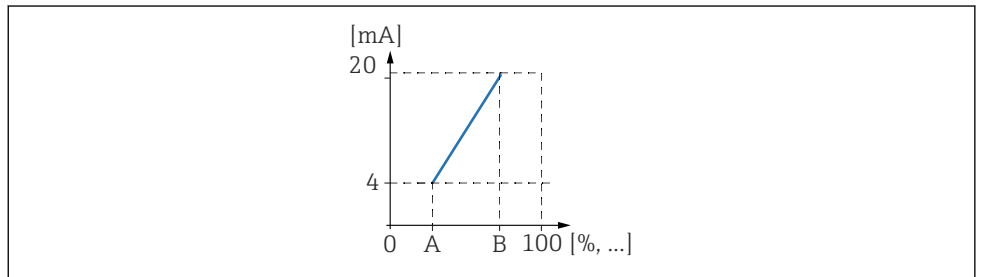
69 电流量程比工作原理
