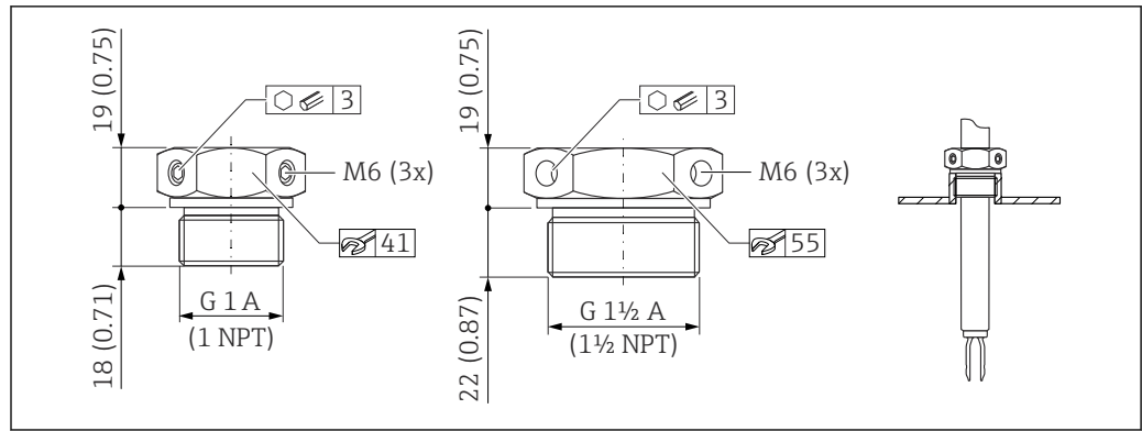
图 25 常压滑动套管 p_e = 0 bar (0 psi)。测量单位 mm (in)
