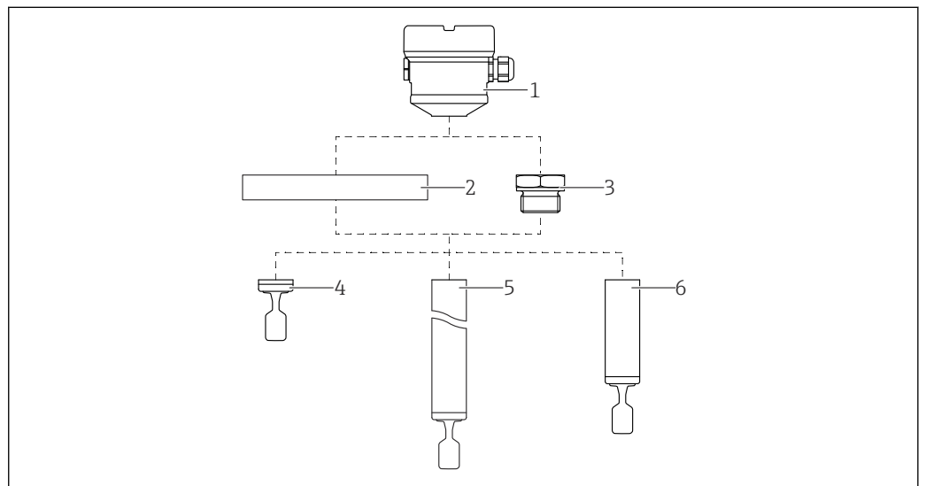
图 1 产品设计
