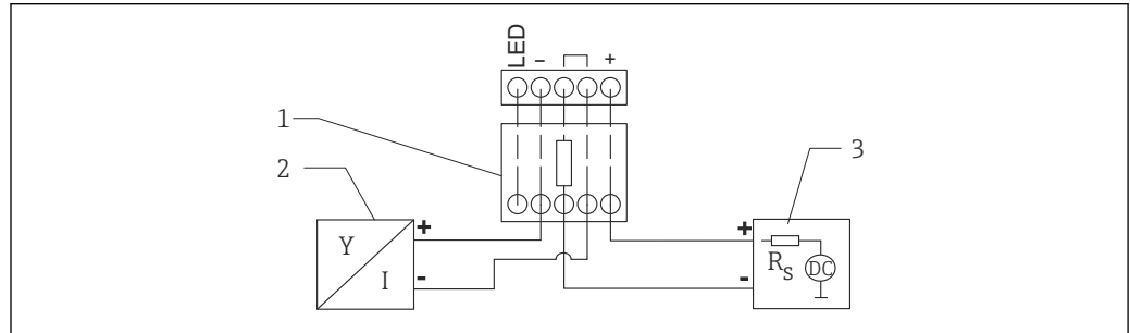
图 4 接线示意图：仪表连接安装有 HART 通信电阻的 RIA15（无背光显示）
