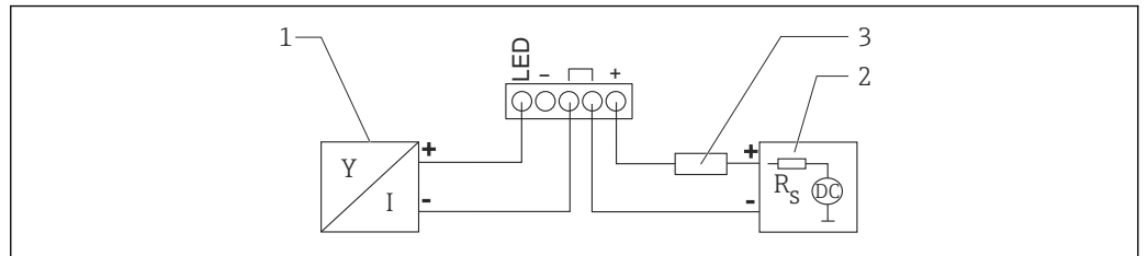
3 接线示意图：HART 通信型仪表连接 RIA15（带背光显示）
