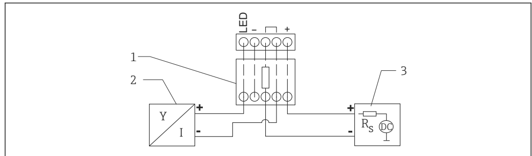
图 5 接线示意图：仪表连接安装有 HART 通信电阻的 RIA15（带背光显示）
