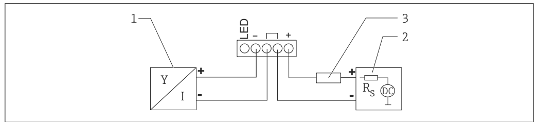
2 接线示意图：HART 通信型仪表连接 RIA15（无背光显示）
