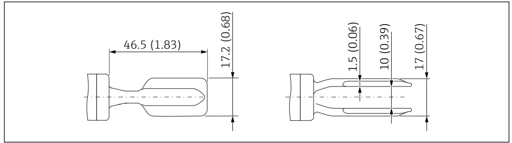
图 27 音叉，带搪瓷涂层。测量单位 mm (in)
