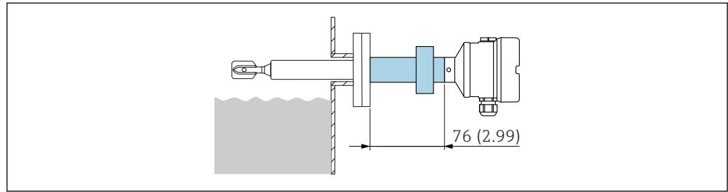
图 24 隔爆玻璃馈通（搭配延长管使用）。测量单位 mm (in)
