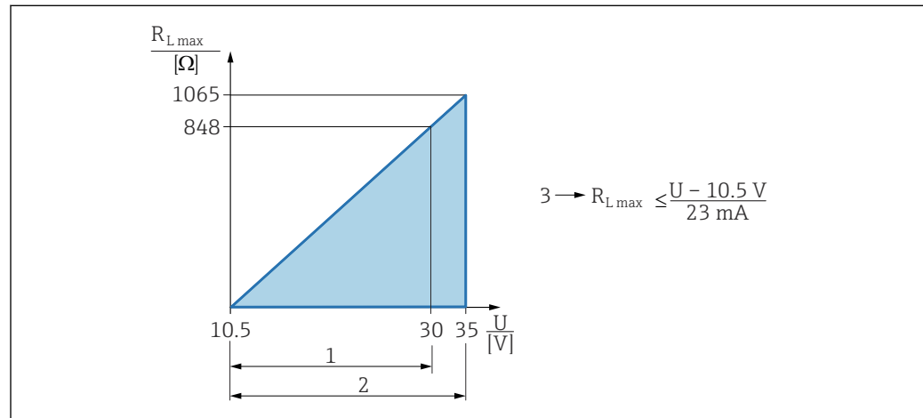
图 2 4 ... 20 mA HART 负载
