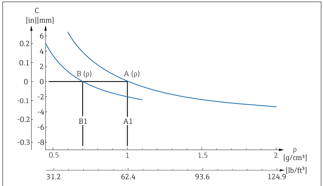
图 8 参考开关点与过程介质密度之间的关系（塑料涂层 (ECTFE、PFA)）
