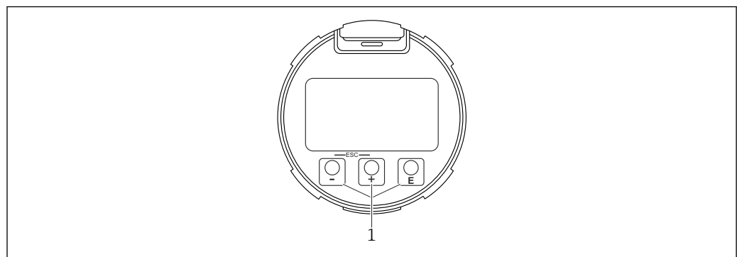
图 30 图形显示单元，带光敏按键（1）
