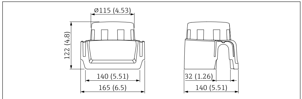
图 32 防护罩，适用单腔体铝外壳。测量单位 mm (in)
