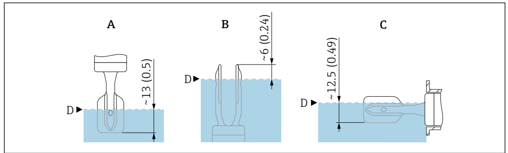
图 6 塑料涂层叉体的常见开关点 (ECTFE、PFA)。测量单位 mm (in)
