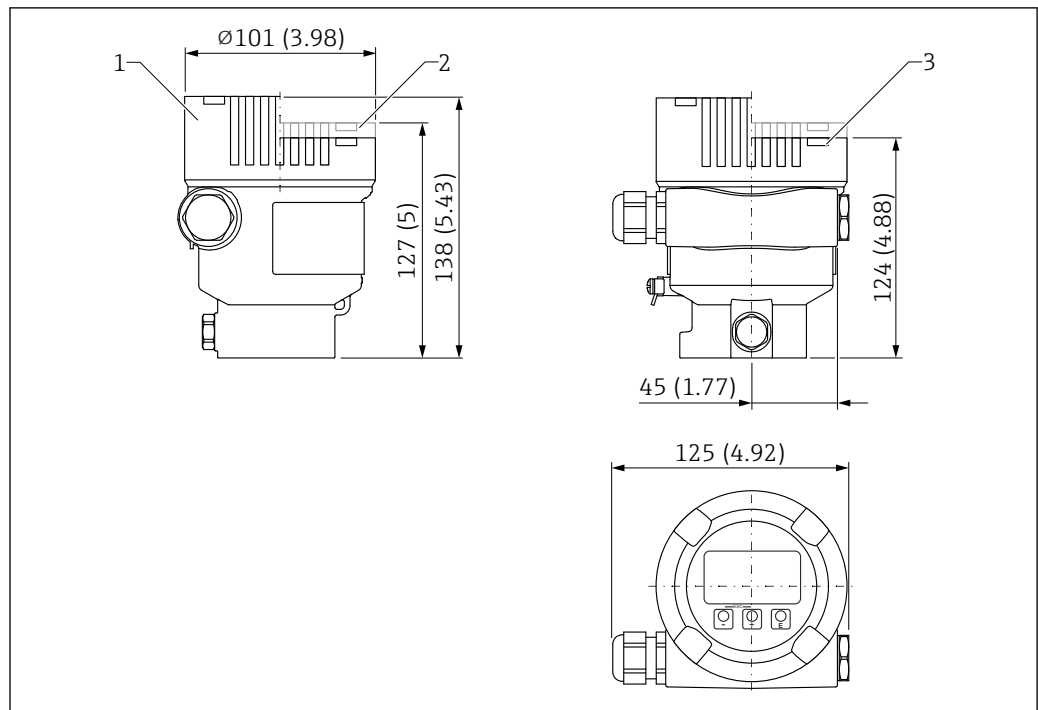
图 22 单腔室铝外壳的外形尺寸示意图。测量单位 mm (in)
