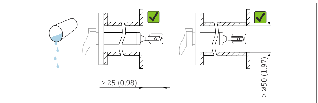
图 11 安装实例: 测量低粘度液体。测量单位 mm (in)
