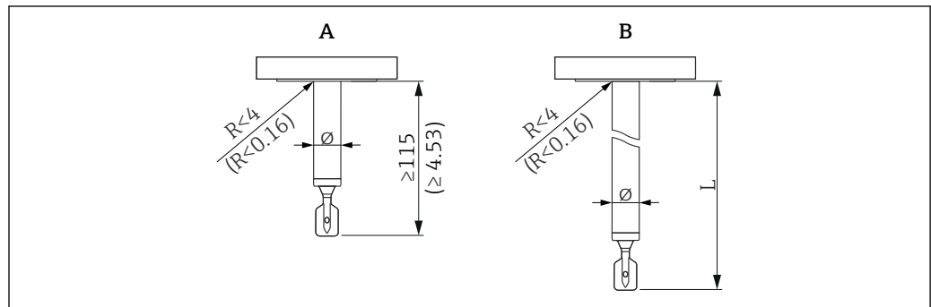
图 25 探头类型：短管型，延长管型。测量单位 mm (in)
