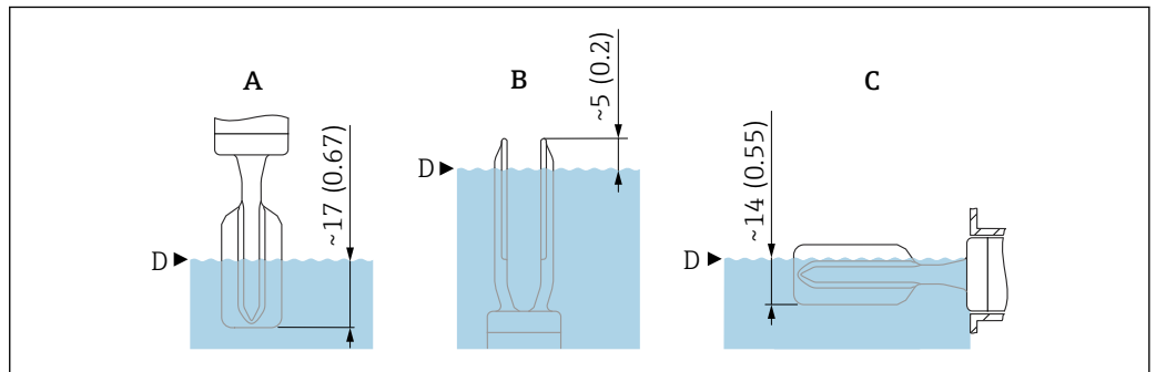
图 7 搪瓷涂层叉体的常见开关点。测量单位 mm (in)
