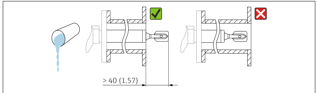
图 12 安装实例：测量高粘度液体。测量单位 mm (in)
