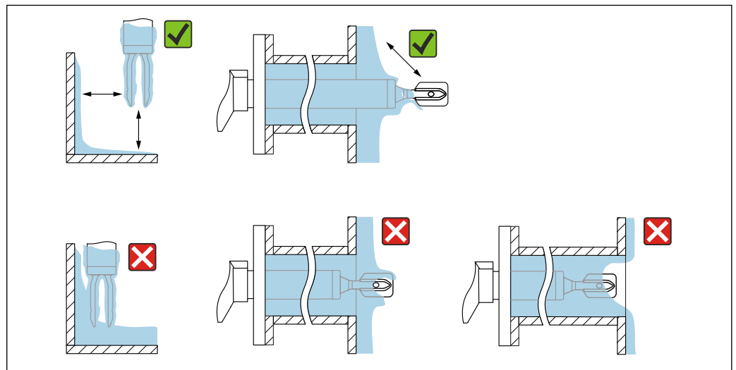
图 13 安装实例：测量高粘度过程介质
