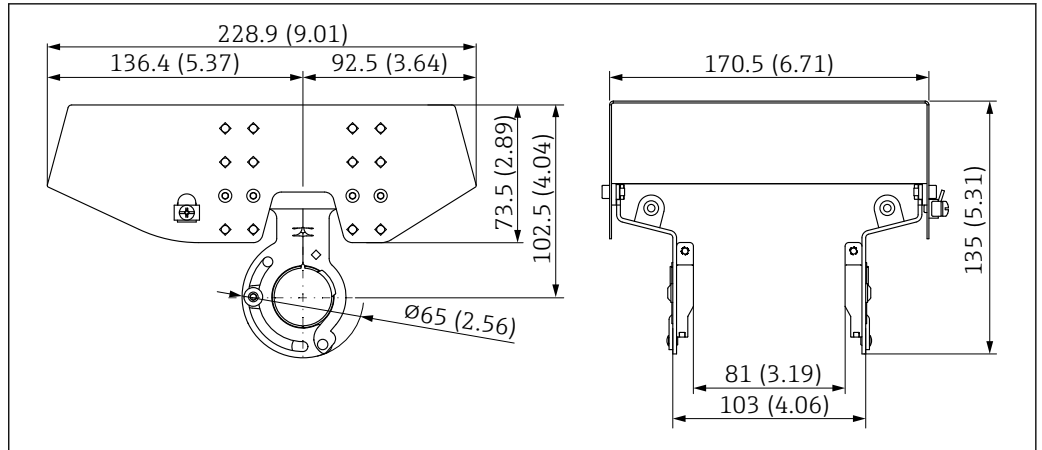
图 31 防护罩，适用双腔体外壳。测量单位 mm (in)
