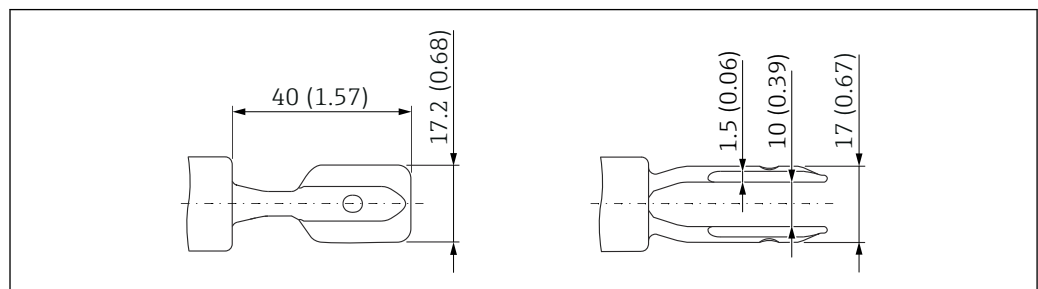
图 26 音叉，带塑料涂层（ECTFE、PFA）。测量单位 mm (in)
