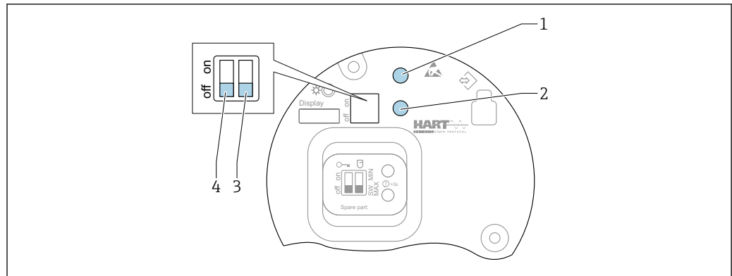
图 29 FEL60H 电子插件上的操作按键和 DIP 开关
