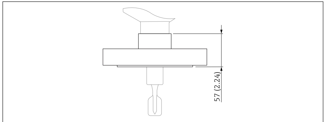
图 28 法兰过程连接（最大高度规格）。测量单位 mm (in)
