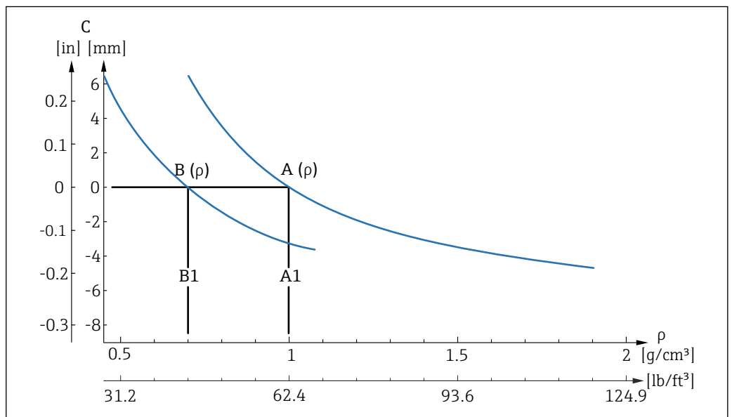
图 9 参考开关点与过程介质密度之间的关系（搪瓷涂层）
