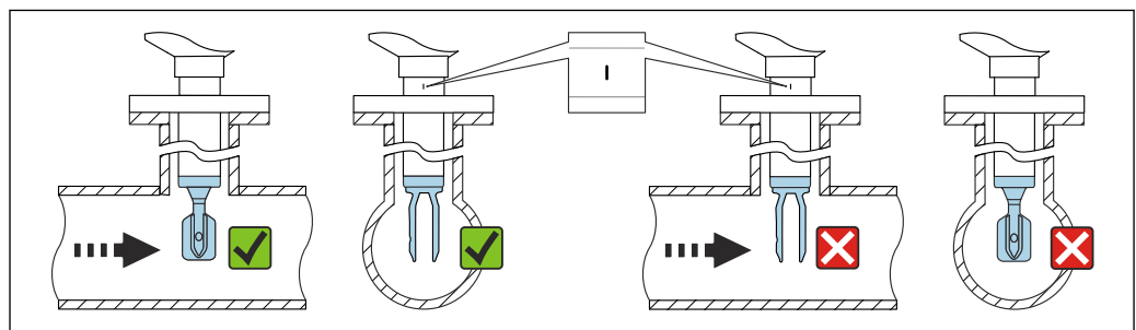
图 16 安装在管道中（注意叉体安装位置和标记）
