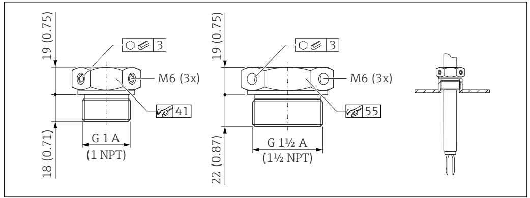
图 37 常压活动套管 p_e = 0 bar (0 psi)。测量单位 mm (in)
