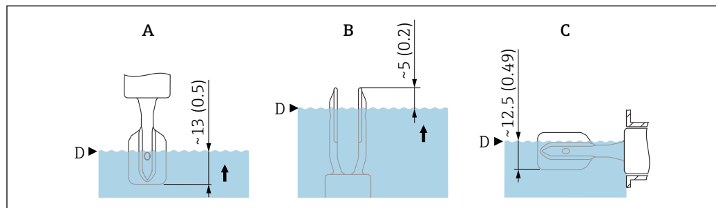
图 6 常见开关点。测量单位 mm (in)
