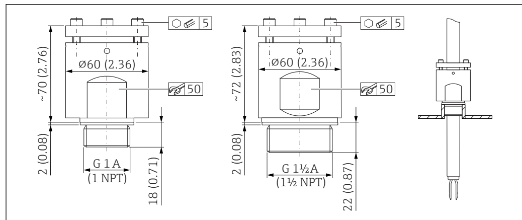
▣ 65 高压滑动套管。测量单位 mm (in)
