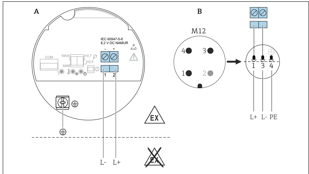
图 13 电子插件 FEL68: 两线制连接, NAMUR 信号 ( \geq 2.2 \text{ mA} / \leq 1.0 \text{ mA} )
