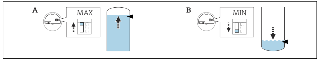
图 54 电子插件上的高限 (MAX) /低限 (MIN) 检测开关位置
