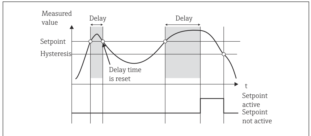
图 10 回差和延迟时间启用
