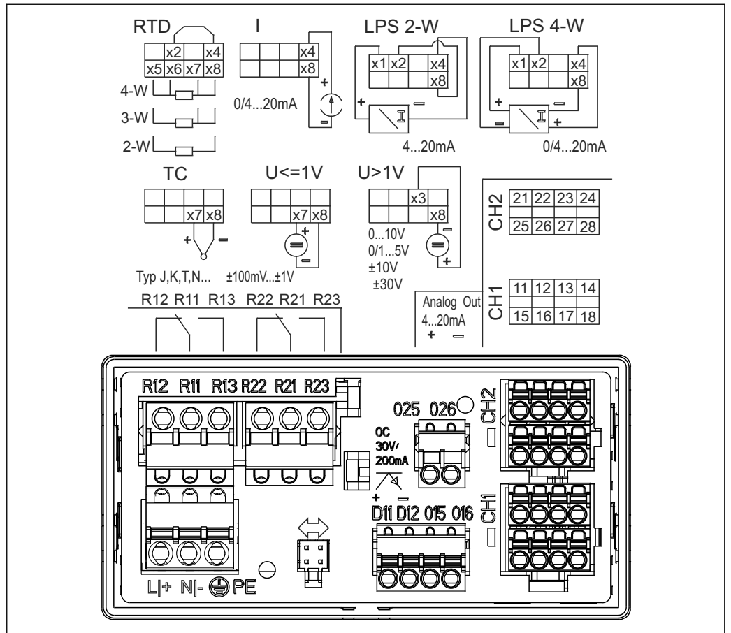
图 13 过程显示仪的接线端子分配 (继电器 (接线端子 Rx1...Rx3) 和通道 2 (接线端子 21...28 和 O25/O26), 可选); 注: 图示为发生电源故障时的继电器触点位置。
