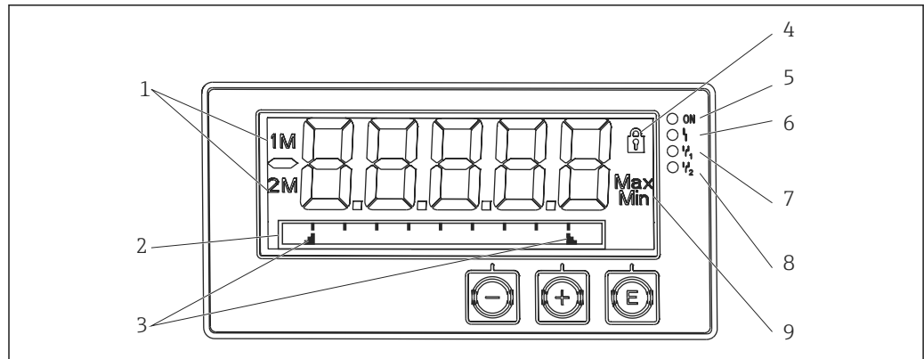
图 3 过程显示仪的显示屏
