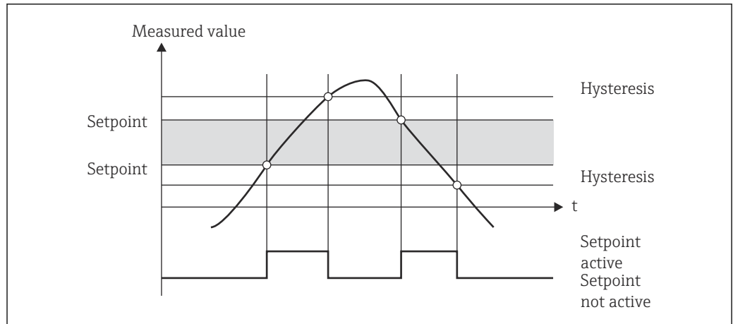
图 8 OutBand 工作模式
