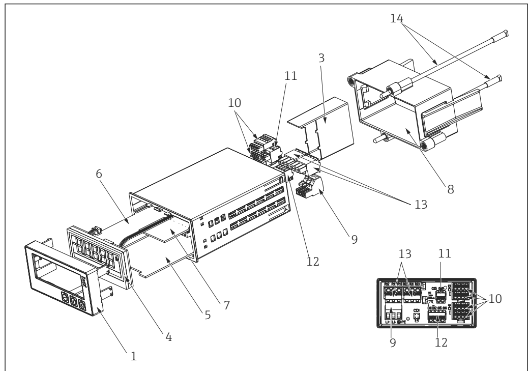
图 12 备件
