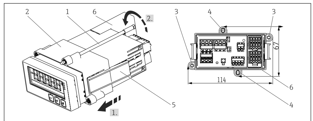
图 1 安装在面板上
