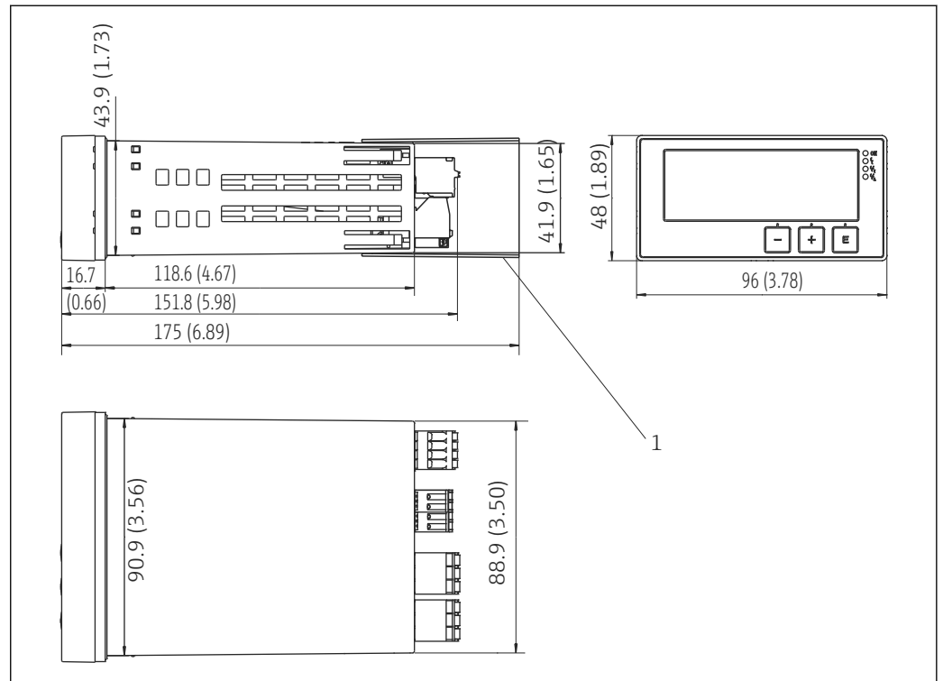
图 14 面板仪表的外形尺寸，单位：mm (in)
