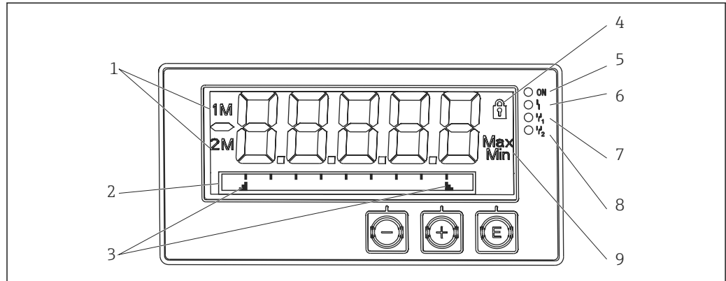
图 15 面板仪表显示屏
