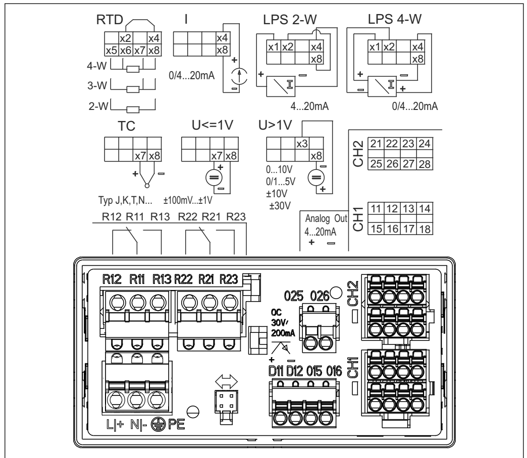
图 2 设备的接线端子分配（通道 2 和继电器，可选）；注：图示为发生电源故障时的继电器触点位置。
