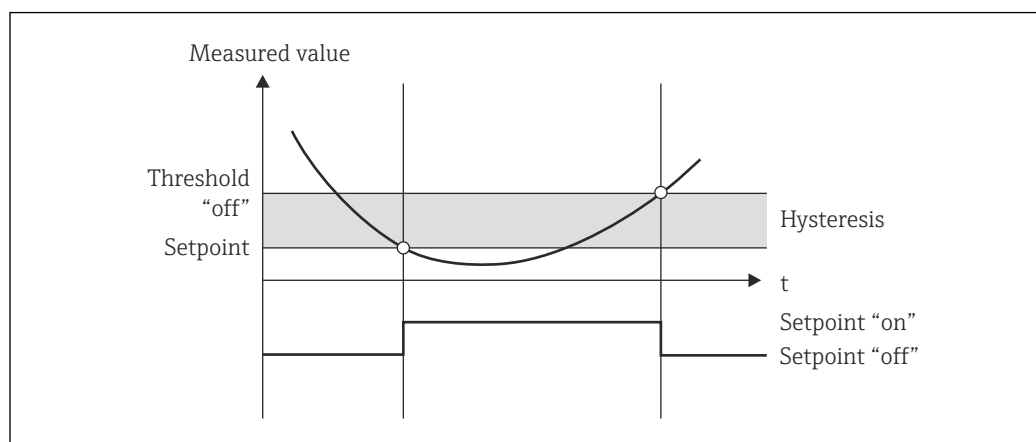
图 5 Min 工作模式
