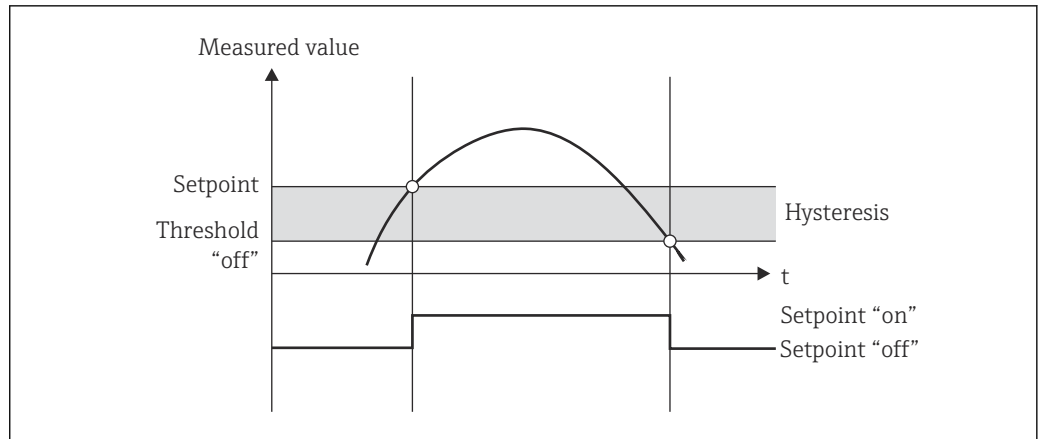
图 6 Max 工作模式
