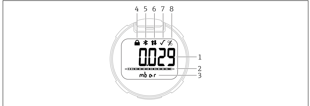
图 9 段码显示屏
