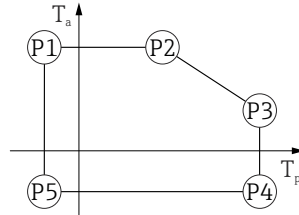
图 10 塑料外壳; 过程温度范围: -10 \dots +150 \text{ }^\circ\text{C} ( +14 \dots +302 \text{ }^\circ\text{F} )
