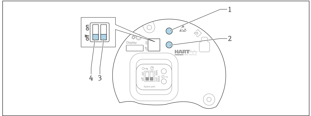
图 56 HART 电子插件上的操作按键和 DIP 开关
