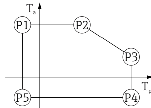
图 23 铝外壳, 带涂层; 过程温度范围: -10 \dots +200 \text{ }^\circ\text{C} ( +14 \dots +392 \text{ }^\circ\text{F} )
