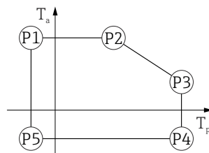
18 塑料外壳; 过程温度范围: -40 ... +150 °C (-40 ... +302 °F)
