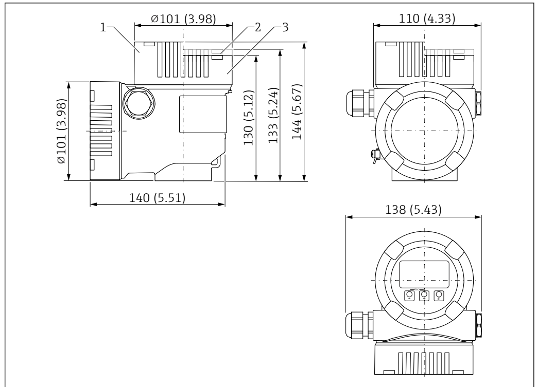
图 44 双腔体外壳 (L 型) 的外形尺寸示意图。测量单位 mm (in)
