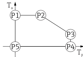
17 塑料外壳; 过程温度范围: 0 ... +200 °C (+32 ... +392 °F), 适用 CSA C/US 认证型仪表
