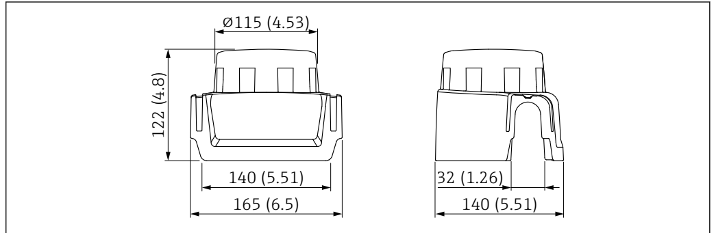
59 外形尺寸示意图。测量单位 mm (in)
