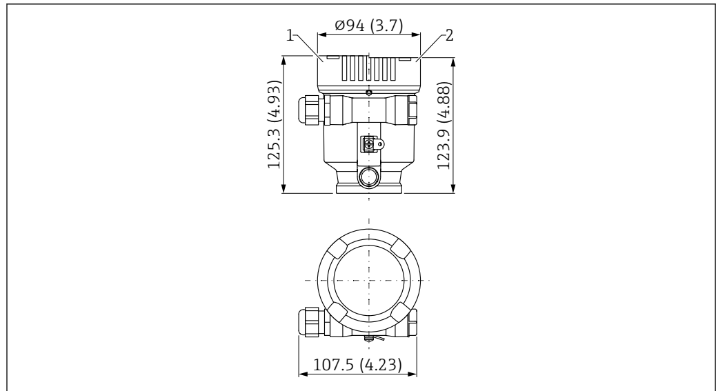
图 40 单腔体塑料 (PBT) 外壳的外形尺寸示意图。测量单位 mm (in)
