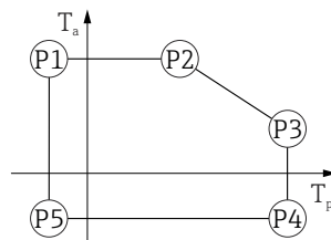
图 24 铝外壳, 带涂层; 过程温度范围: -20 \dots +150 \text{ }^\circ\text{C} ( -4 \dots +302 \text{ }^\circ\text{F} )
