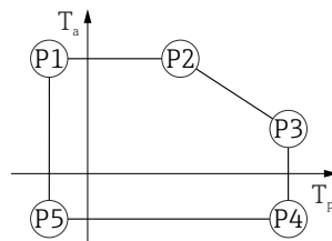
图 12 塑料外壳; 过程温度范围: -10 \dots +200 \text{ }^\circ\text{C} ( +14 \dots +392 \text{ }^\circ\text{F} )
