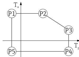
☐ 36 316L 外壳, 卫生型; 过程温度范围: -20 ... +150 °C (-4 ... +302 °F)
